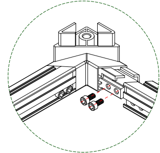
A : 2 Way Connector
