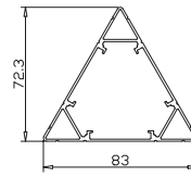
120° pole 3912#
